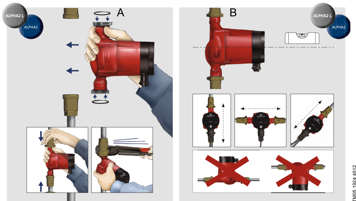
Фиг. 3 Монтаж на GRUNDFOS ALPHA2 L
